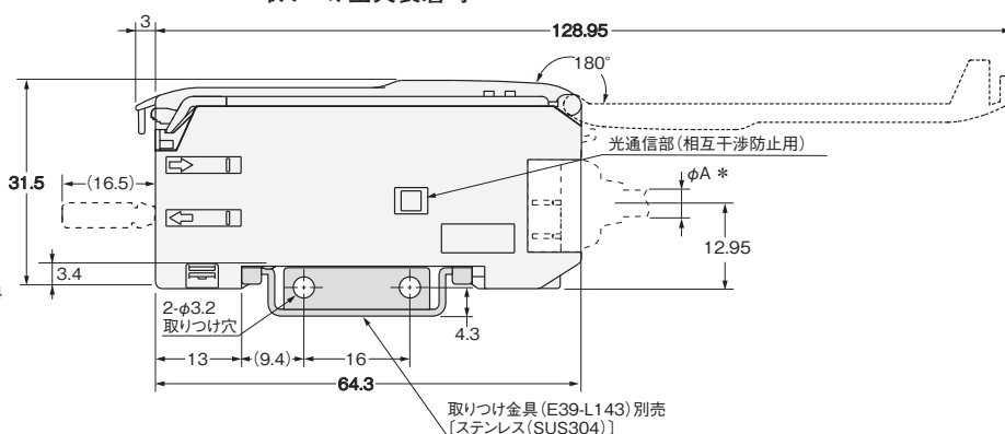
取り付け金具装着時
