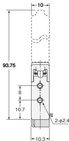
取り付け穴加工寸法
