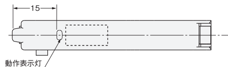
DINレール装着時
