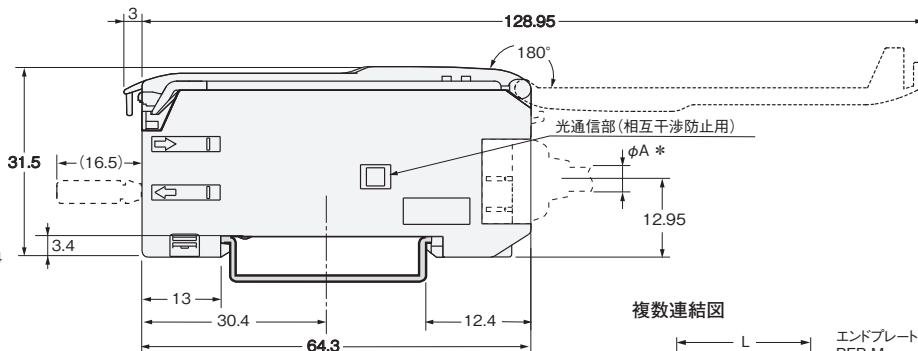
DINレール装着時
