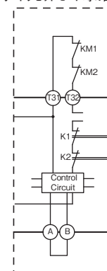
オートリセットモード時の配線
