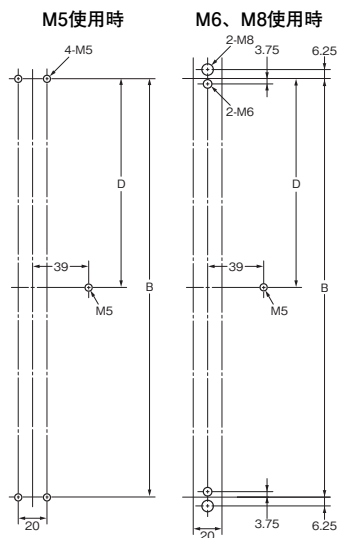
取付穴加工寸法
