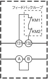
オートリセットモード時の配線
