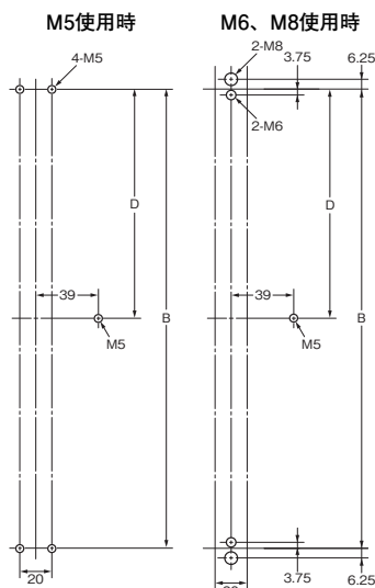
取付穴加工寸法
