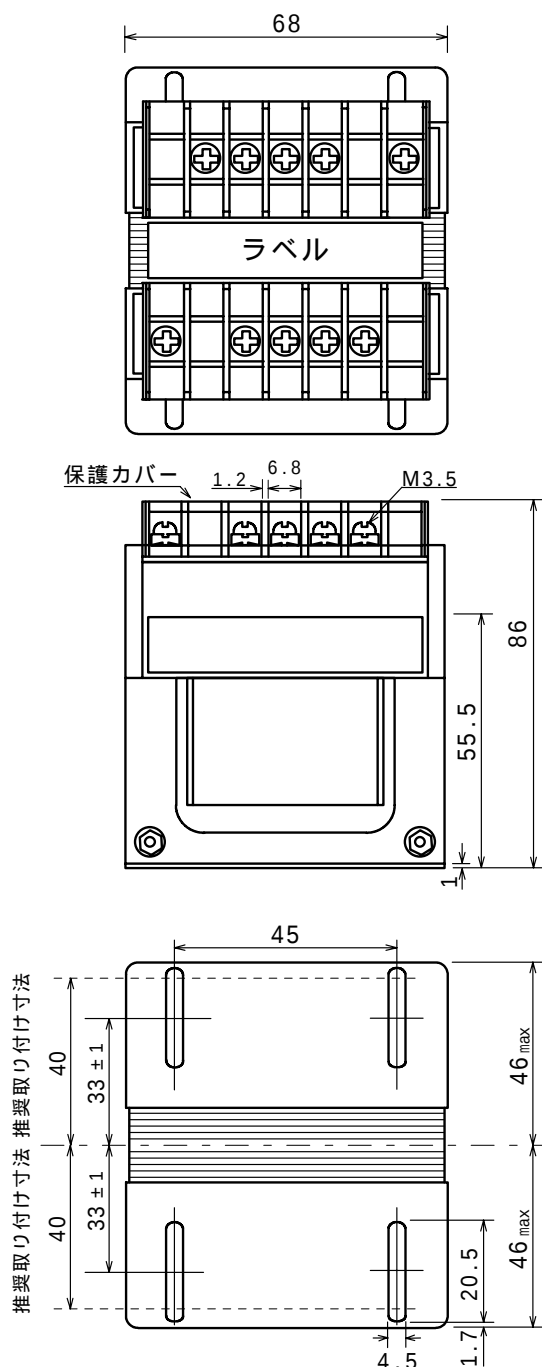
(单位 mm)
