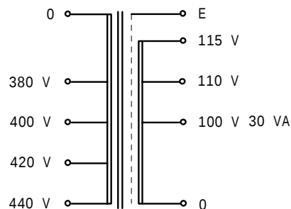
結線図
