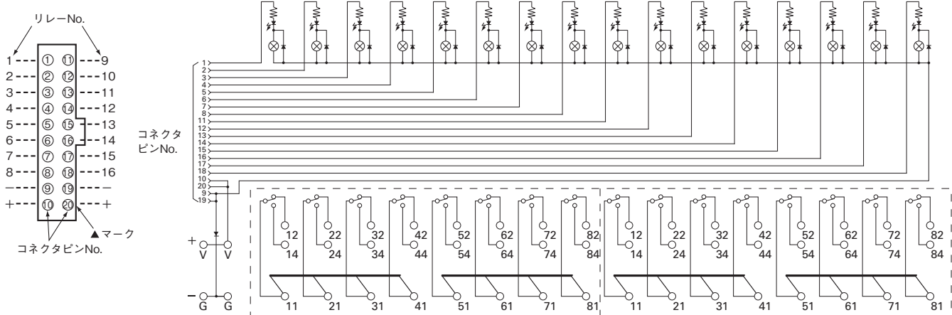
コネクタピン配置図 (TOP VIEW)
