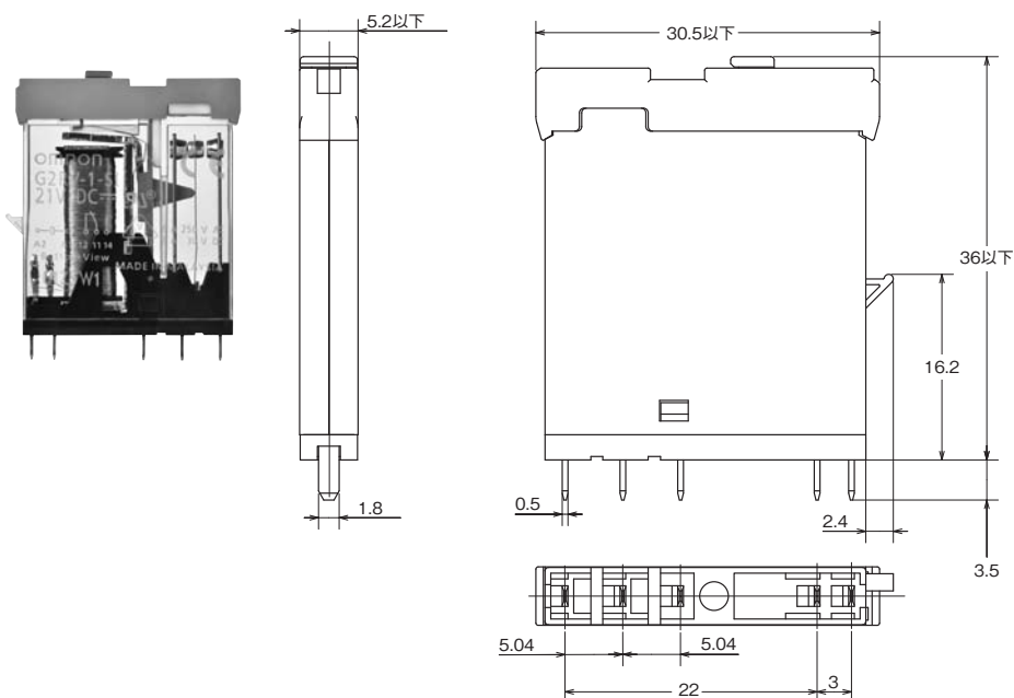
端子配置/内部接続図 (TOP VIEW)
