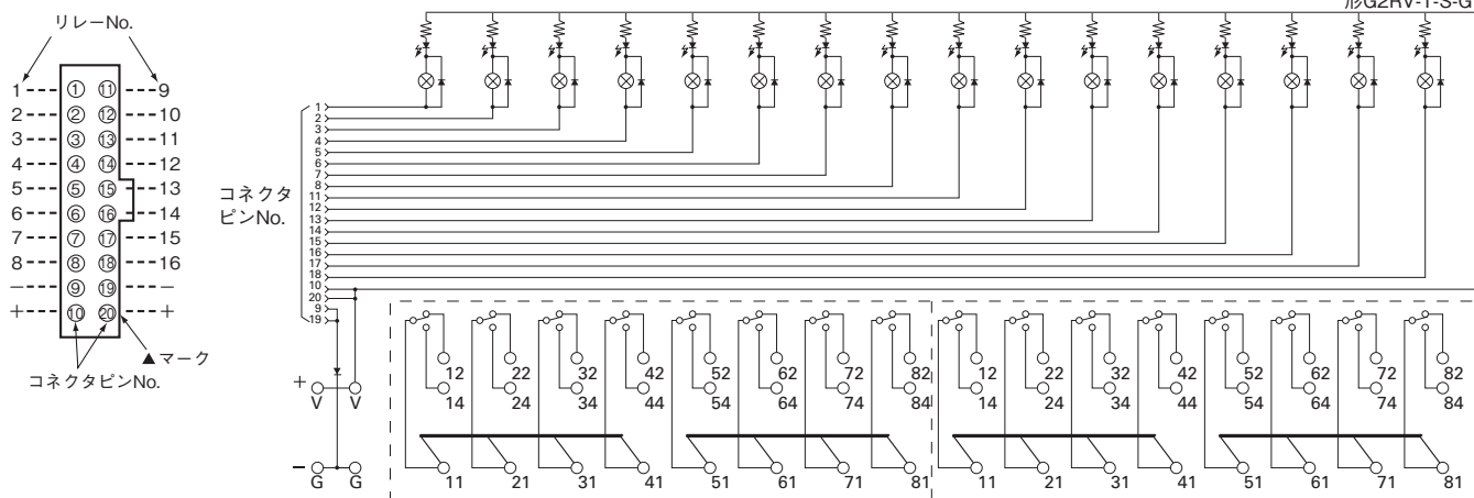
コネクタピン配置図 (TOP VIEW)
