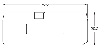
形XW5E-P2.5-2.2-1
