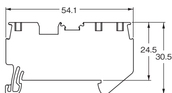
形XW5T-P1.5-1.2-1 (BL) / 形XW5G-P1.5-1.2-1
