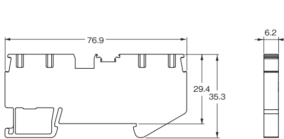
形XW5T-P4.0-2.2-1 (BL) / 形XW5G-P4.0-2.2-1
