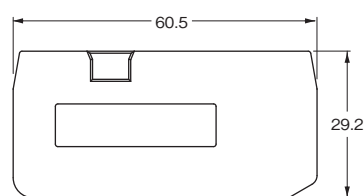
形XW5E-P2.5-1.1-2
