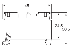
形XW5T-P1.5-1.1-1 (BL) / 形XW5G-P1.5-1.1-1
