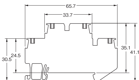
形XW5T-P2.5-1.2-1 (BL) / 形XW5G-P2.5-1.2-1
