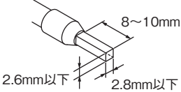
フェルール端子の加工寸法
