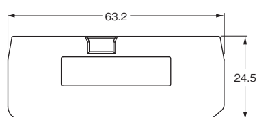
形XW5E-P2.5-1.1-1
