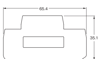
形XW5E-P1.5-1.1-2
