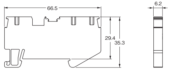
形XW5T-P4.0-1.2-1 (BL) / 形XW5G-P4.0-1.2-1
