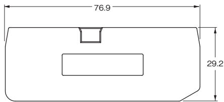
形XW5Z-EP6(ストッパ)
