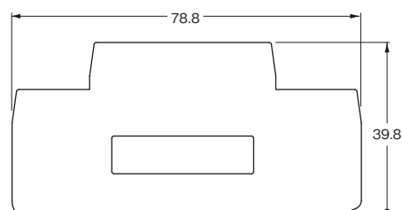
形XW5E-P2.5-1.1-2
