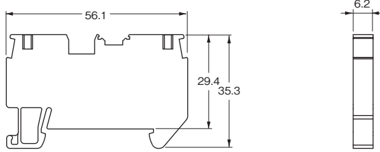
形XW5T-P4.0-1.1-1 (BL) / 形XW5G-P4.0-1.1-1
