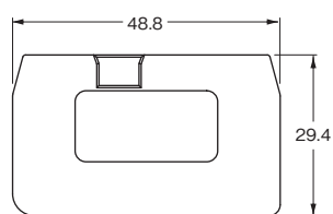
形XW5E-P2.5-2.2-1
