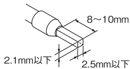
フェルル端子の加工寸法
