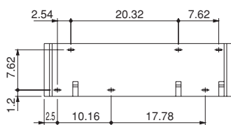
※背面図
