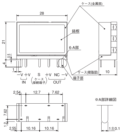
※背面図
