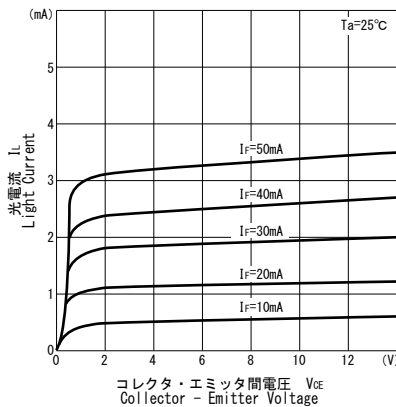
■光電流/コレクタ・エミッタ間電圧特性 I_L/V_{CE}
