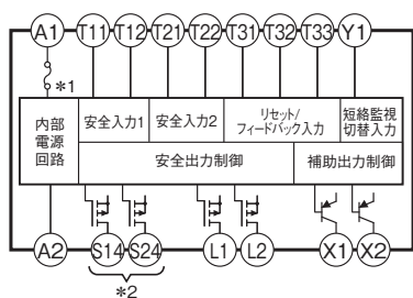
形G9SX-BC202-□(単機能ユニット)
