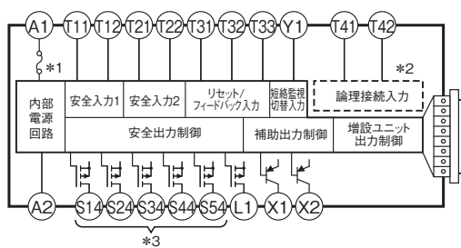
形G9SX-AD322-□(高機能ユニット)
