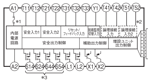
形G9SX-ADA222-□(高機能ユニット)
