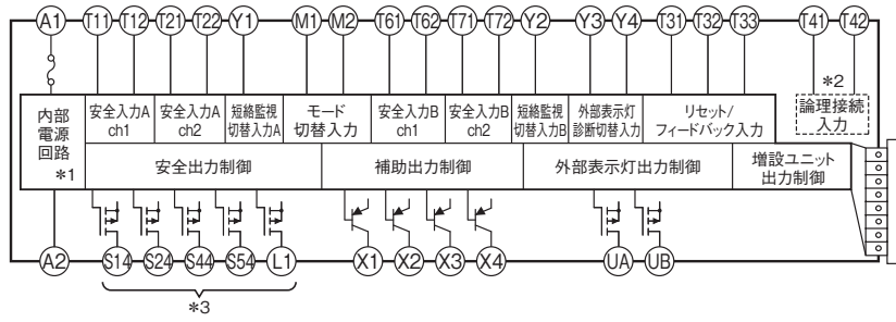
形G9SX-GS226-T15-□ (セーフティガード・スイッチングユニット)
