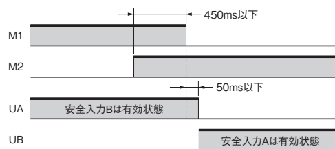
〈M2がON後、M1がOFFする場合〉
