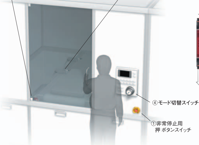
③ セーフティ・リミットスイッチ
