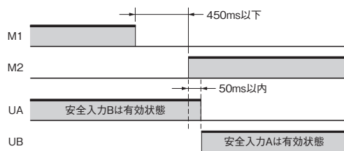
〈M1がOFF後、M2がONする場合〉
