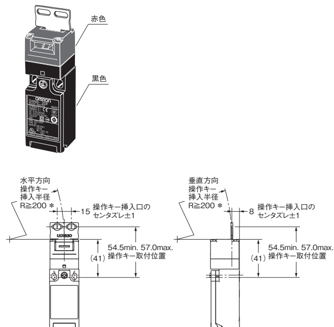
形D4NS-1□F+形D4DS-K1 上面操作キー挿入口使用時
