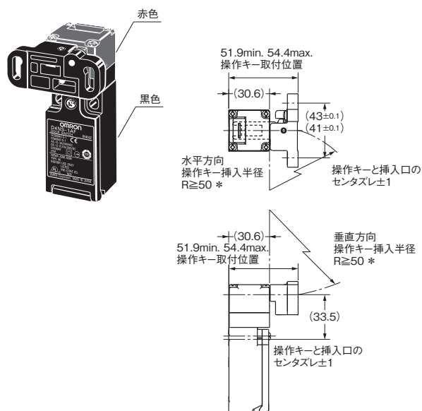
形D4NS-1□F+形D4DS-K5 正面操作キー挿入口使用時
