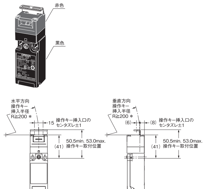
形D4NS-1□F+形D4DS-K2 上面操作キー挿入口使用時
