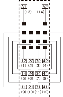
端子配置/内部接続図
