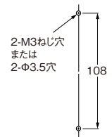
取り付け穴加工寸法
