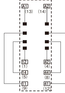
端子配置/内部接続図
