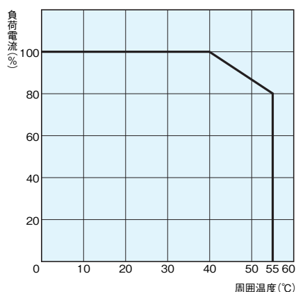
形G3PW-A220E□、形G3PW-A245E□
