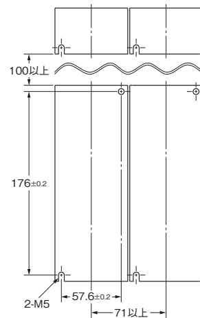
取り付け穴加工寸法
