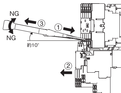
取り外し工具 （形J78KC）
