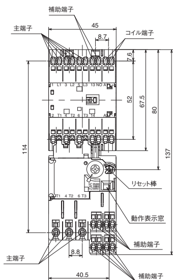
電磁開閉器
