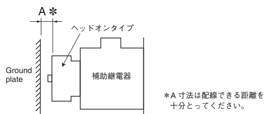
図3. 取り付けスペース
