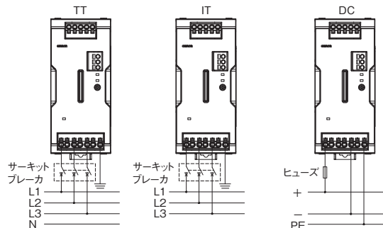
入力の配線 (TT、IT、DC)
