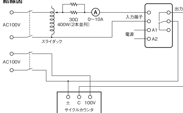
結線図
