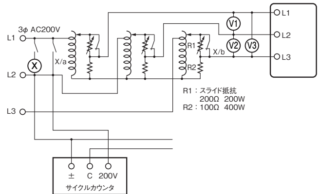
結線図2
