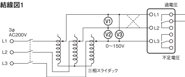
結線図1
