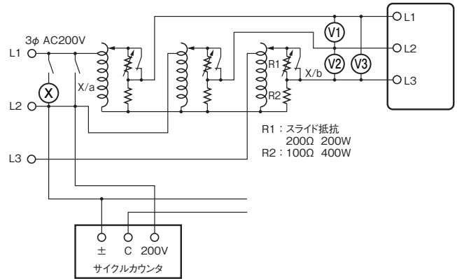
結線図2
