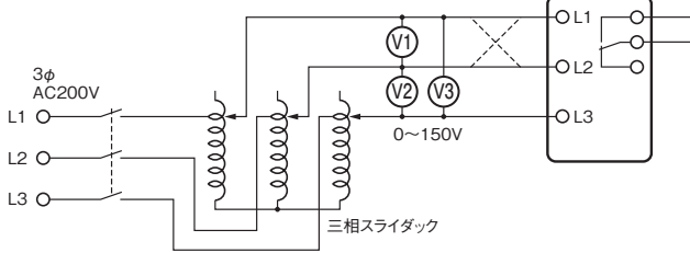
結線図1
