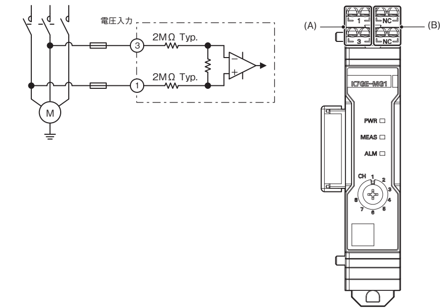
プローブユニット 形K7GE-MG1
