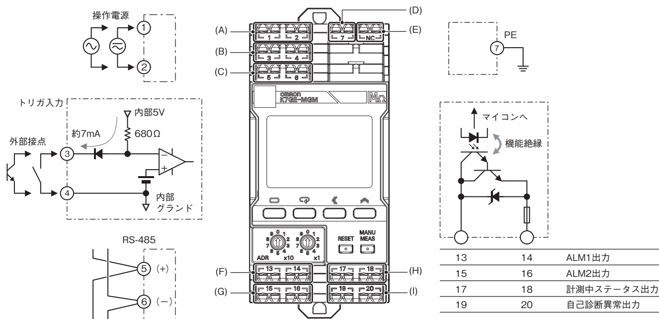
メインユニット 形K7GE-MGM
