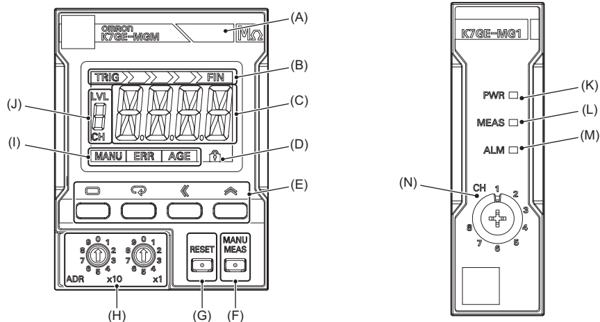
メインユニット 形K7GE-MGM
