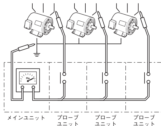
メインユニット (形K7GE-MGM)
