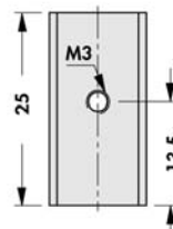
SK 95 25 SOT 32
