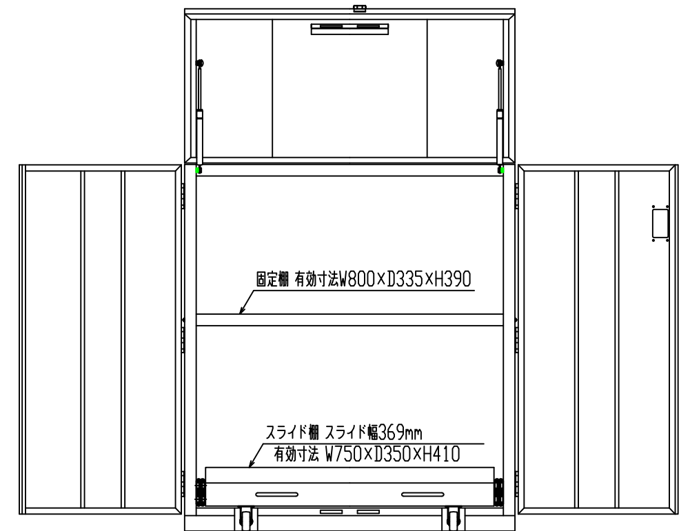
< 扉開放図 >
