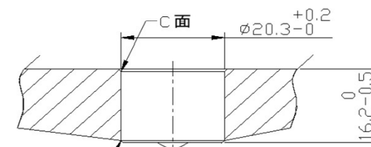
推奨取付穴寸法
