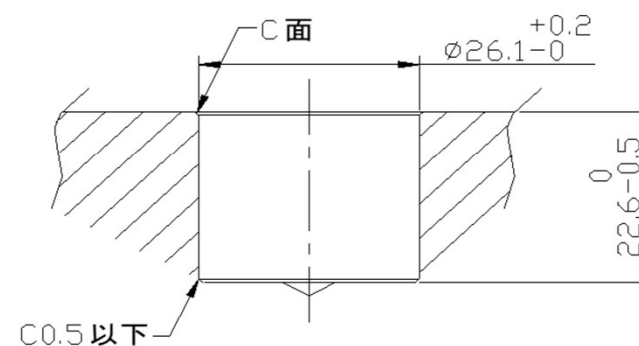
推奨取付穴寸法
