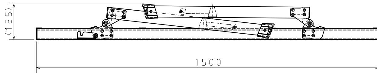
収納寸法
