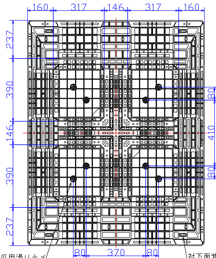
裏面図
