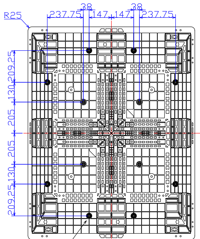
上面図
