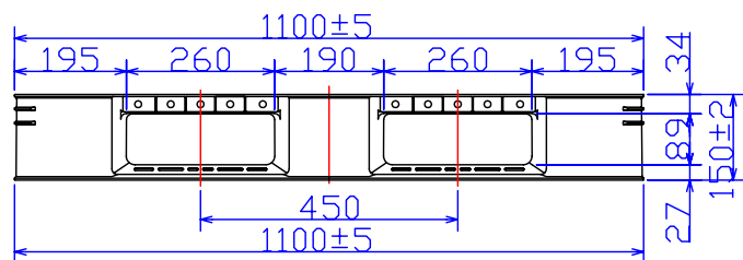
短側面図
