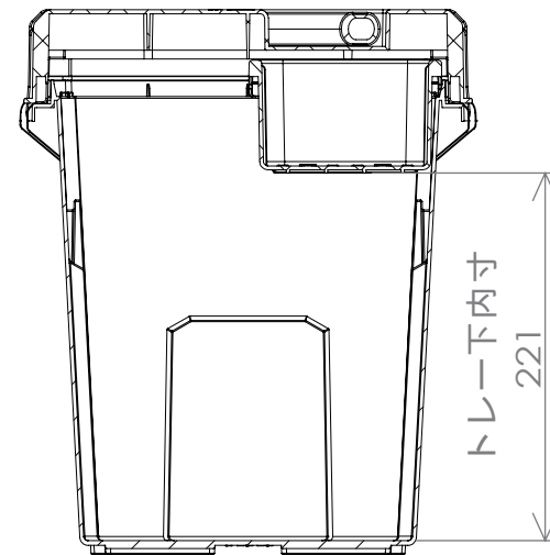
断面図 A-A
