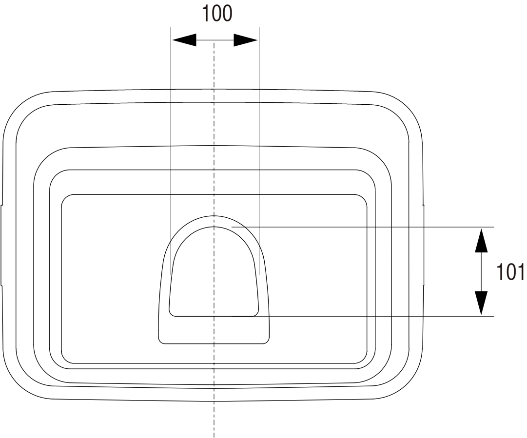
平面視
