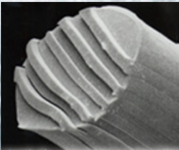
1本の糸が11本に分割された極細割繊維糸
