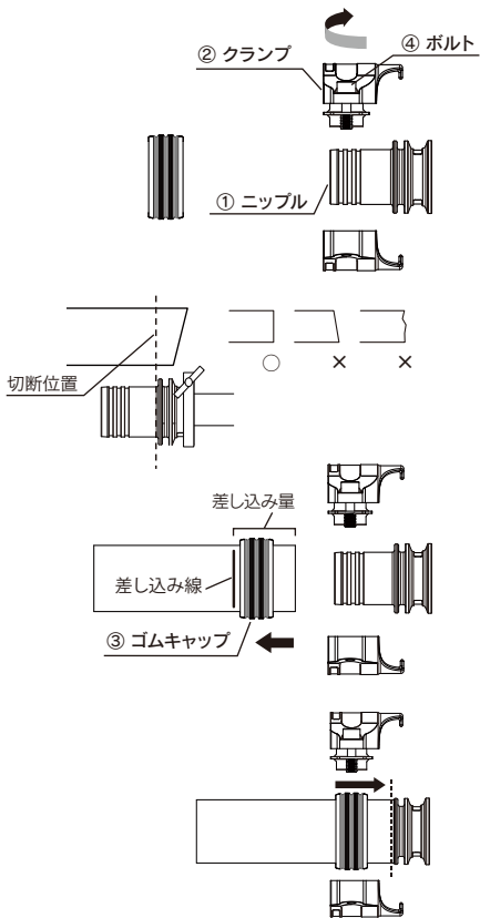
適正なゴムキャップ差し込み量
