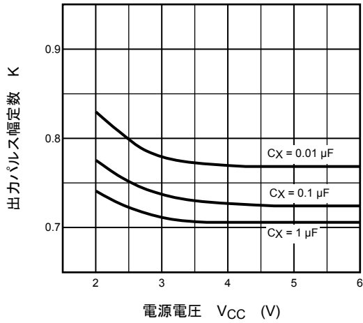
出力パルス幅定数 K - 電源電圧 (標準) (外付け抵抗 (R X ) = 10 kΩ: t wOUT = K · C X · R X )
