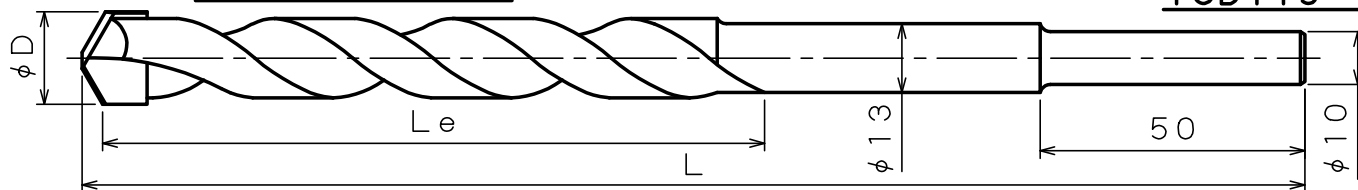
TCD160~TCD220
