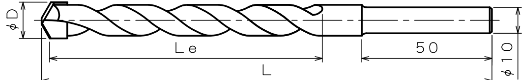
TCD115~TCD150
