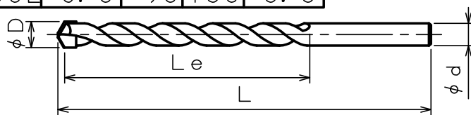
TCD25~TCD110
