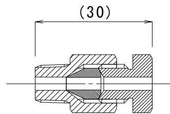
組図 (1:1)
