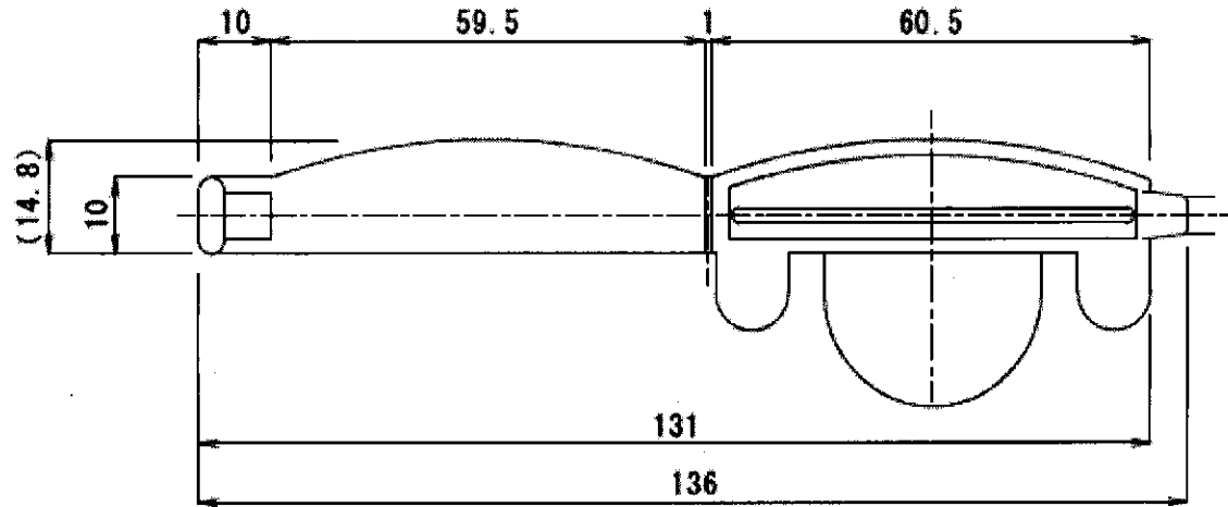
裏面図
