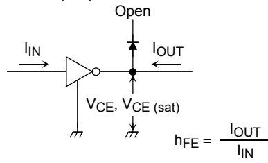
2. V_{CE(sat)} , h_{FE}
