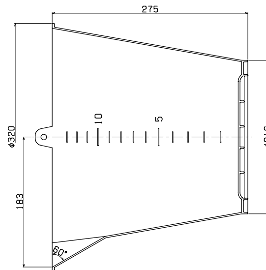
中心断面図
