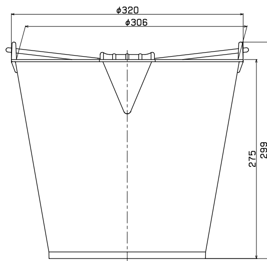
正面図
