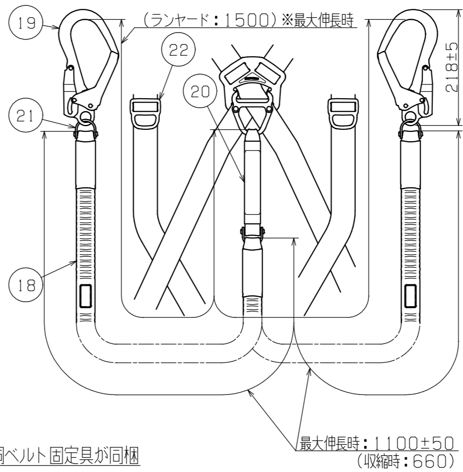
背部D環に伸縮式ランヤード直付け式 100kg以下用
