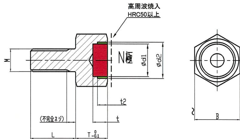
マグネット付六角ボルト焼入タイプ規格表
