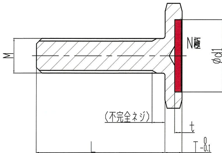
マグネット付六角ボルト低頭タイプ規格表
