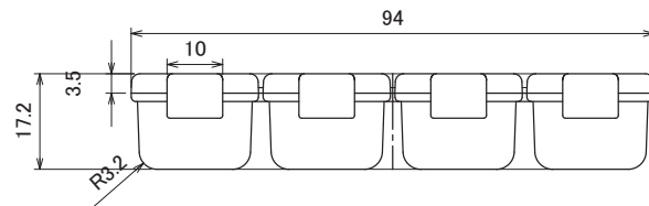
B-B`線断面図
