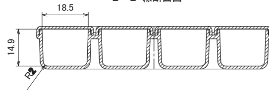
B-B`線断面図
