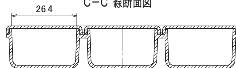
C-C`線断面図
