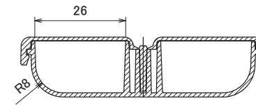
A-A`線断面図
