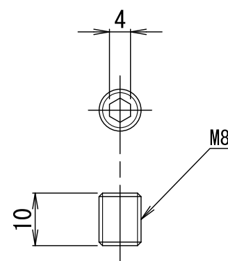
六角穴付き止めねじ：2個
