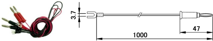
TLA-35 Y字端子⇔バナナプラグ 【半田付け】
