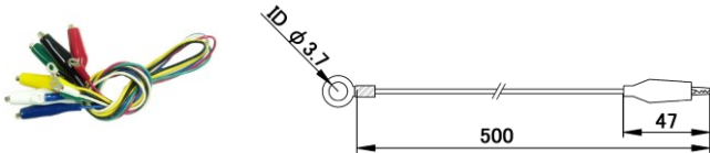
TLA-36 丸端子⇔シールドクリップM 【半田付け】
