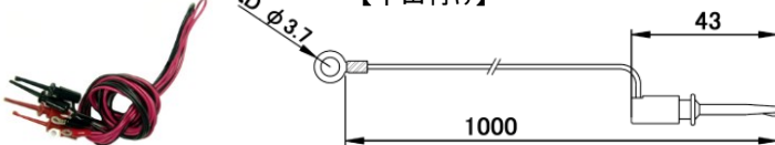
TLA-39 丸端子⇔ICクリップS 【半田付け】
