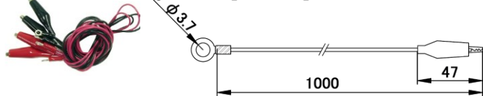
TLA-37 丸端子⇔シールドクリップM 【半田付け】
