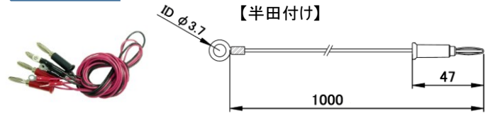
TLA-42 シールドクリップM両端【圧着式】 【半田付け】
