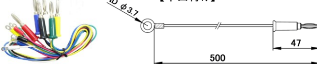
TLA-40 丸端子⇔バナナプラグ 【半田付け】
