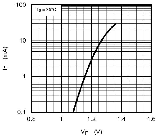
Fig. 13.1.3 I_F - V_F
