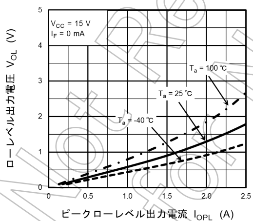
図 13.2.11 V_{OL} - I_{OPL}
