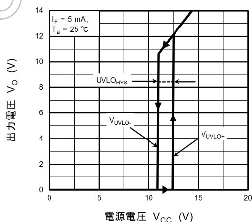
図 13.2.6 V_O(V_{UVLO}) - V_{CC}
