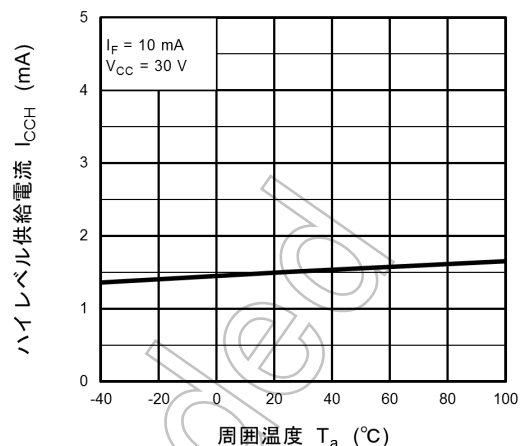
図 13.2.8 I_{CCH} - T_a
