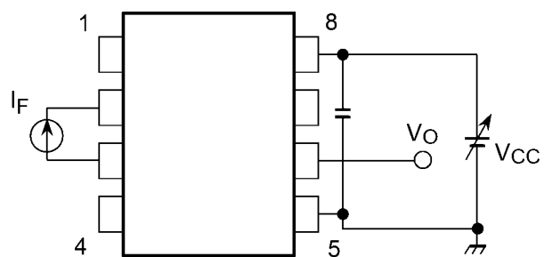
図 13.1.9 V_{CC} - V_O(VUVLO) 測定回路
