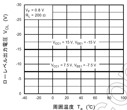
図 13.2.9 V_{OL} - T_a
