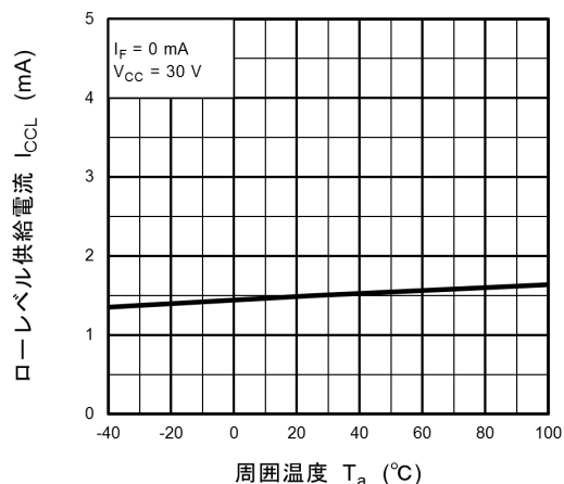
図 13.2.7 I_{CCL} - T_a
