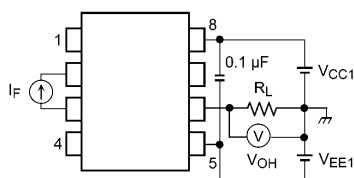
図 13.1.3 V_{OH} 測定回路
