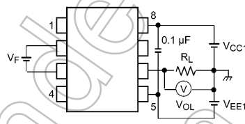
図 13.1.4 V_{OL} 測定回路
