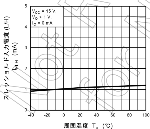
図 13.2.5 I_{FLH} - T_a
