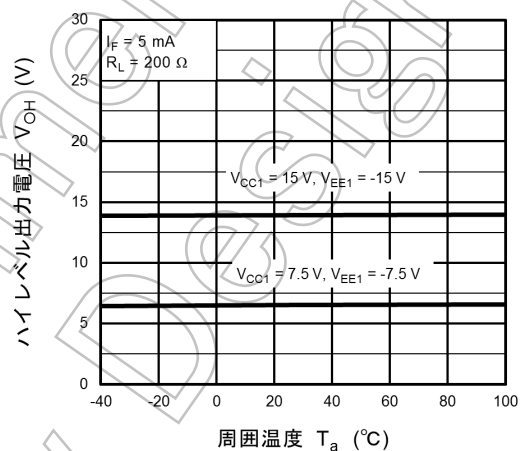
図 13.2.10 V_{OH} - T_a
