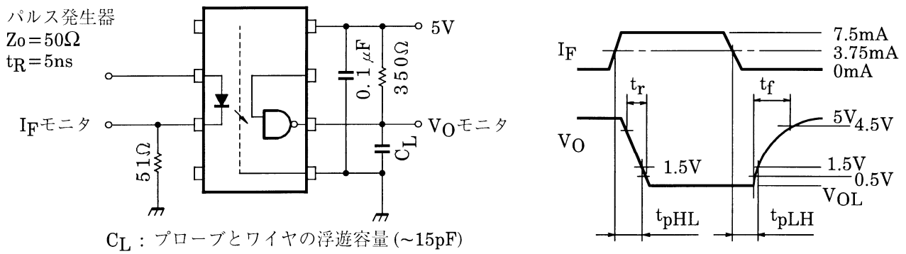
図2 t_{EHL} 、 t_{ELH} 測定回路、波形
