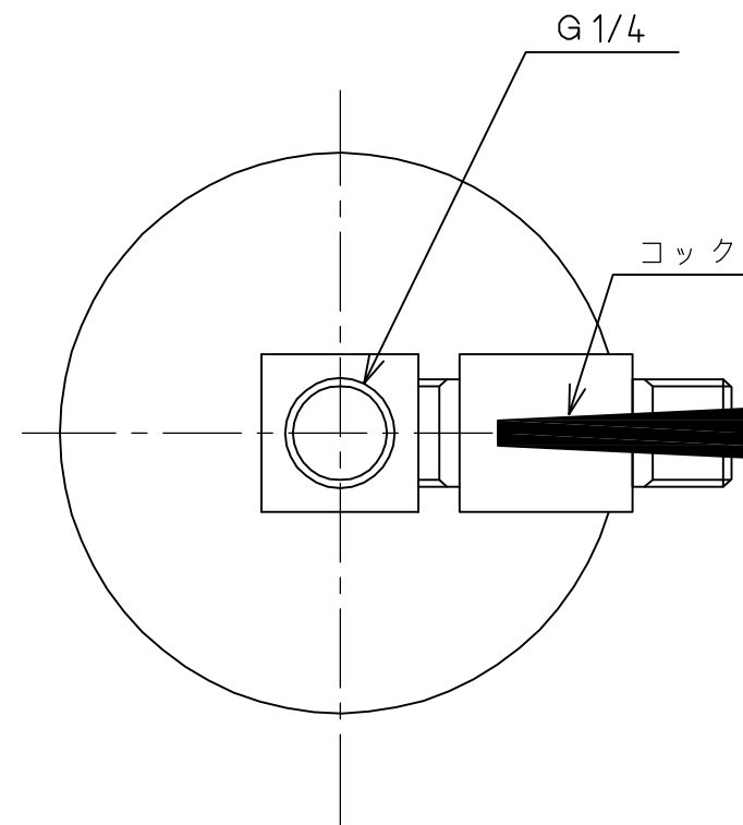
A - A 上面寸法図
