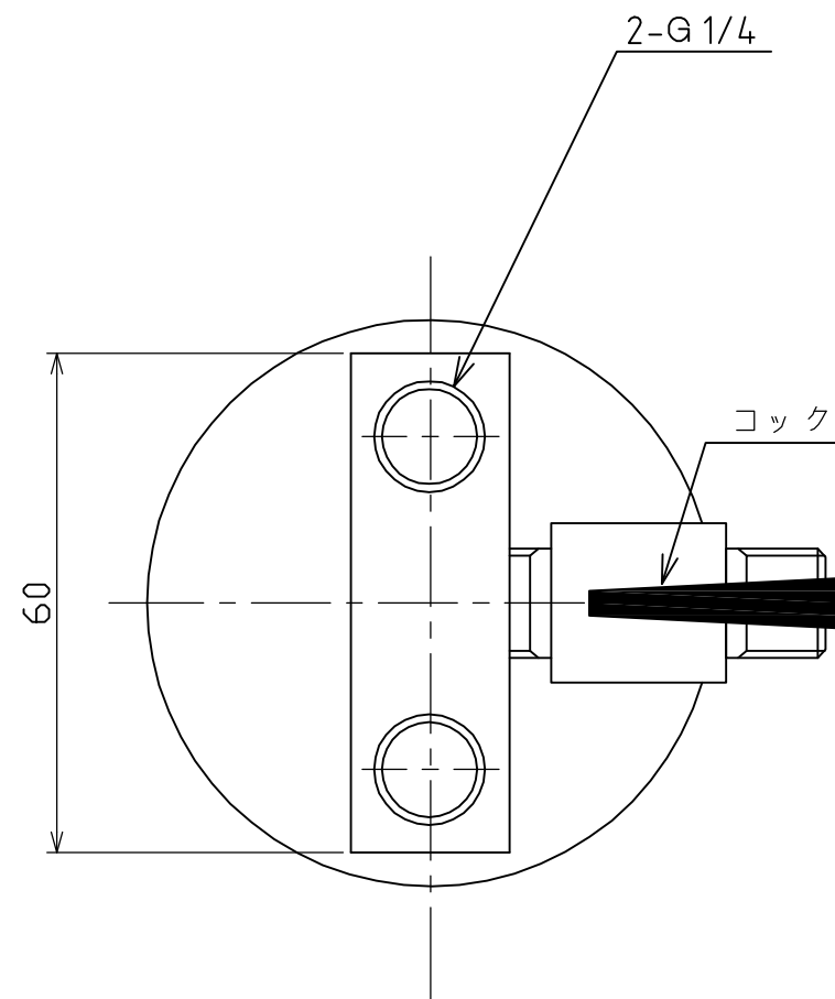
A - A 上面寸法図
