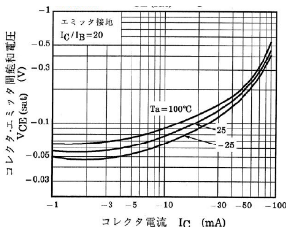
図 10.23 RN2405 V_{CE(sat)}-I_C
