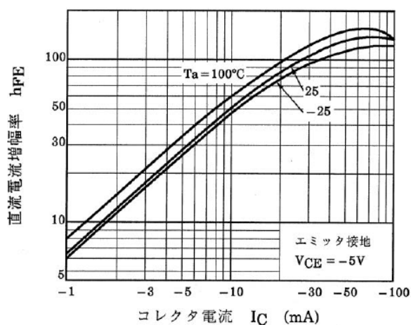
図 10.13 RN2401 h_{FE} - I_C
