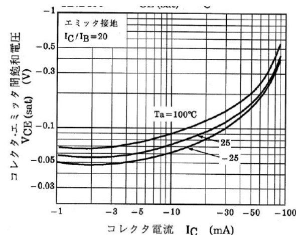
図 10.24 RN2406 V_{CE(sat)}-I_C
