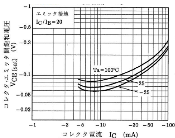
図 10.19 RN2401 V_{CE(sat)}-I_C
