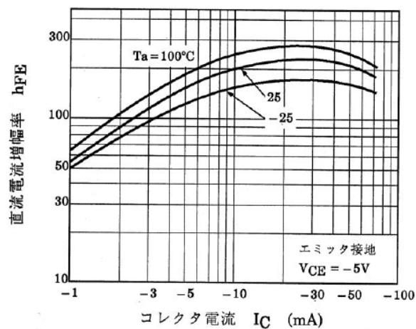
図 10.16 RN2404 h_{FE} - I_C
