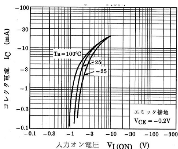
図 10.4 RN2404 I_C - V_{I(ON)}
