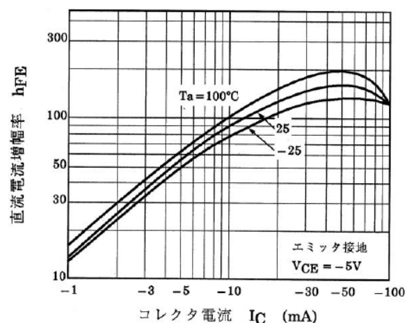
図 10.14 RN2402 h_{FE} - I_C
