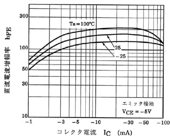
図 10.18 RN2406 h_{FE} - I_C
