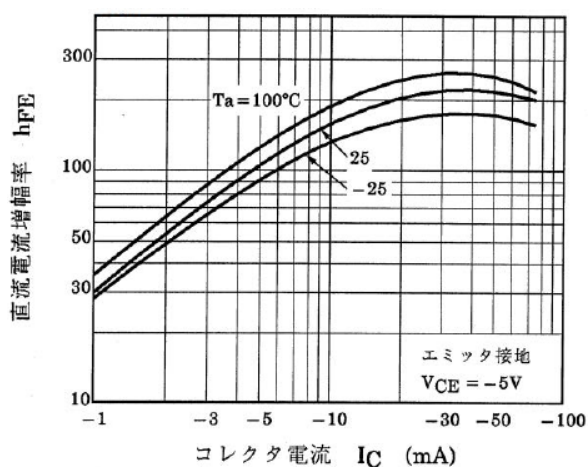
図 10.15 RN2403 h_{FE} - I_C
