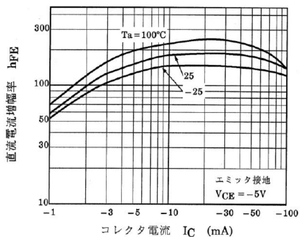
図 10.17 RN2405 h_{FE} - I_C
