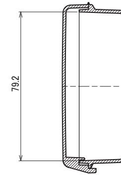
A-A線断面図
