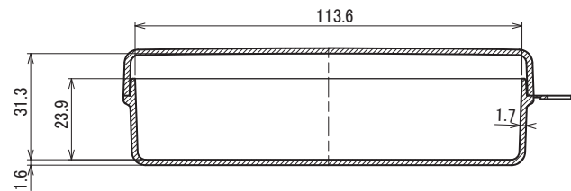
線断面図
