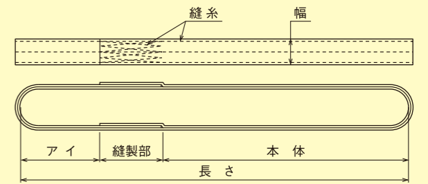
図2 エンドレス形ベルトスリングの例
