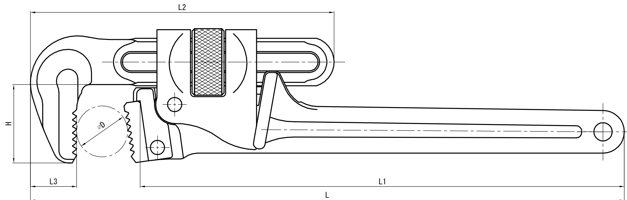
寸法表
